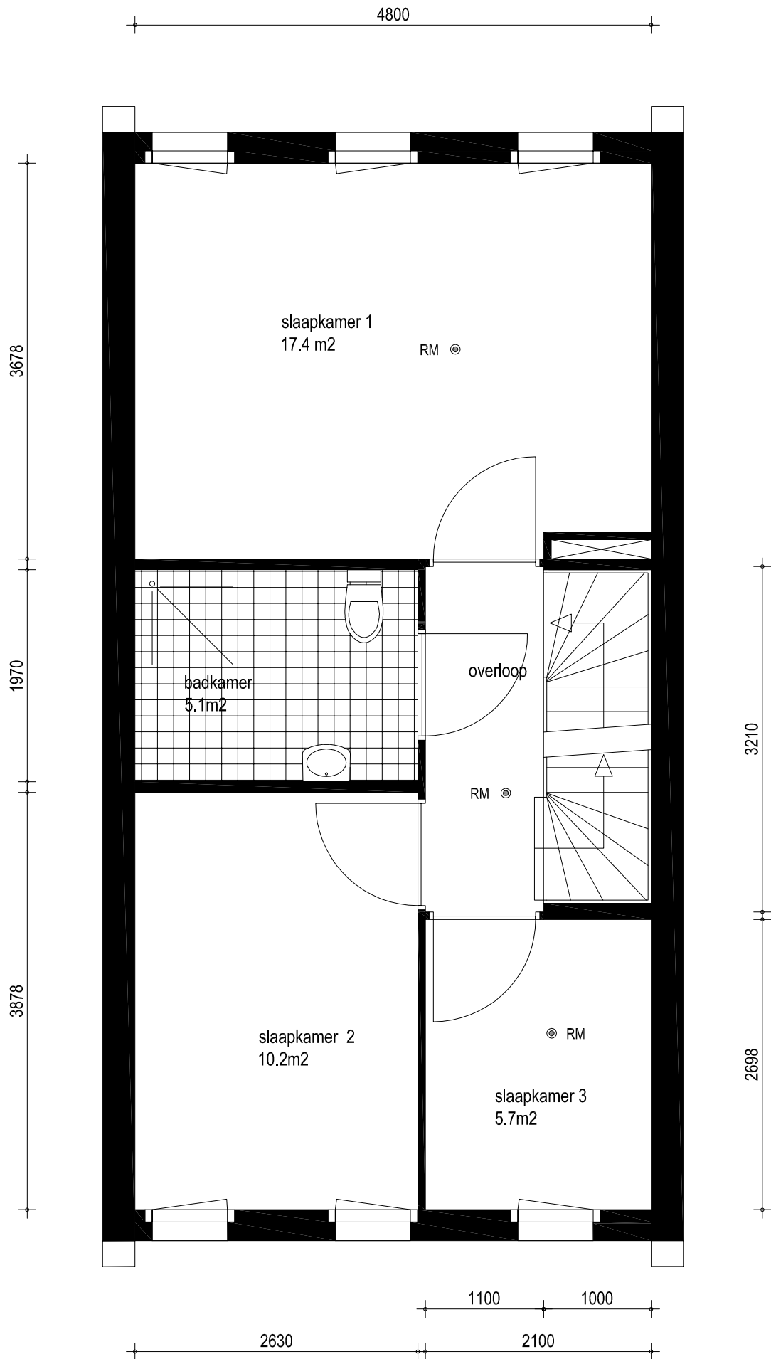
tussenwoning - eerste verdieping
