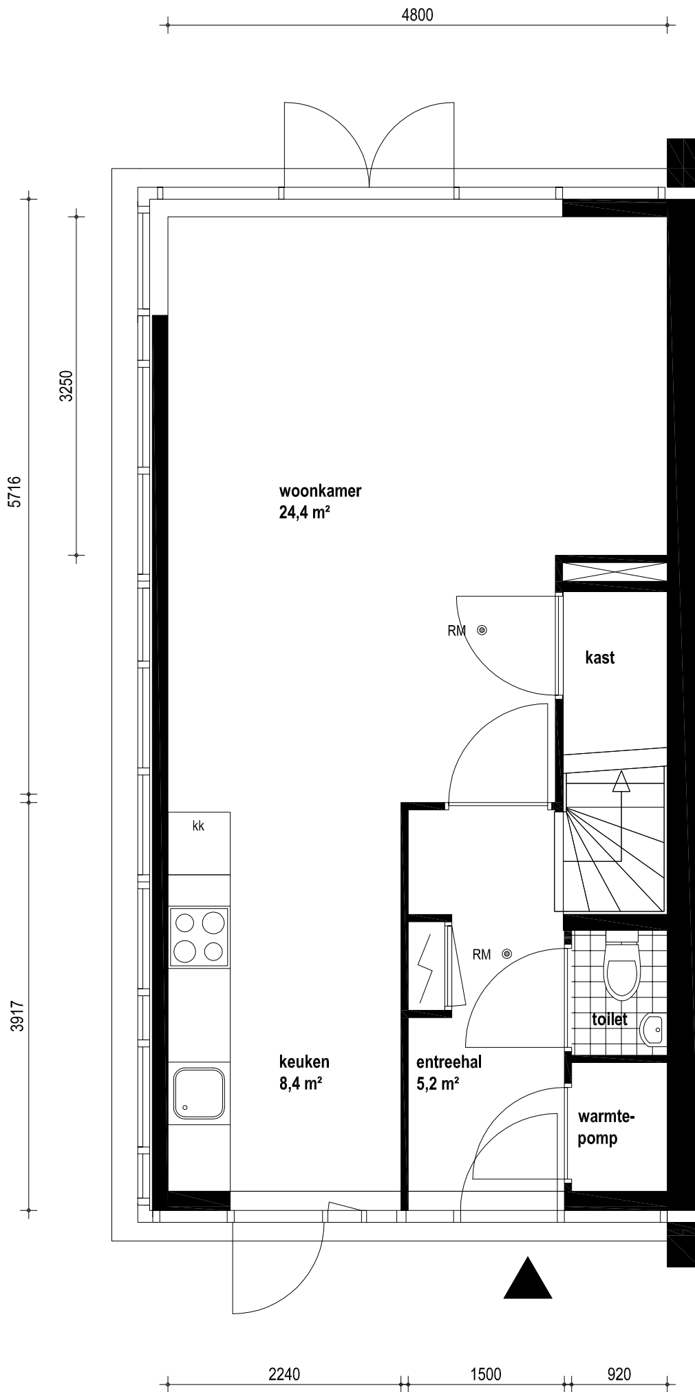
kopwoning - begane grond
