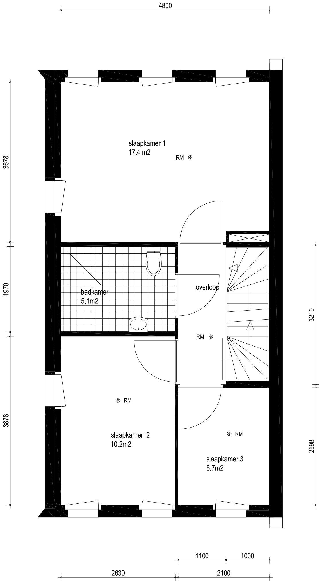
kopwoning - eerste verdieping
